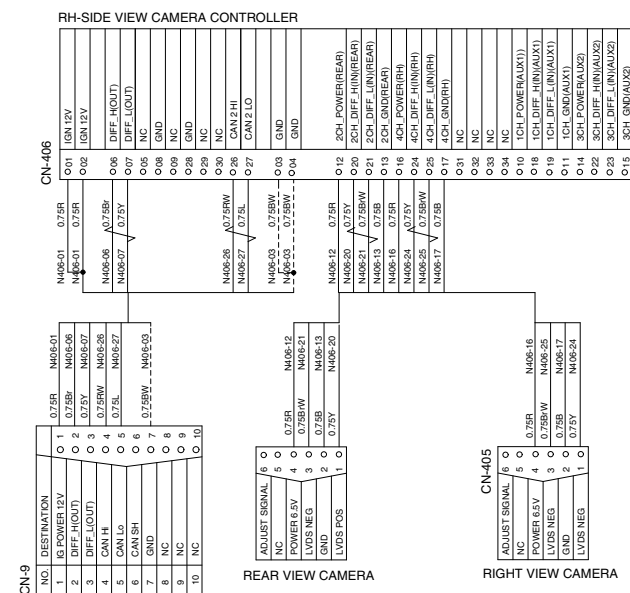
RH MIRROR VIEW SYTEM(EI06)
